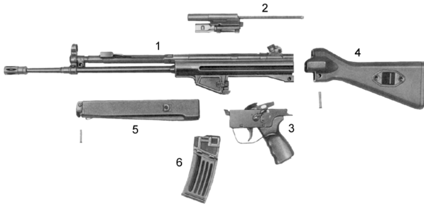
Fig. 6 Assemblies
